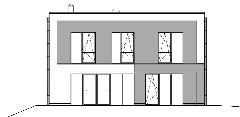
Západní pohled
