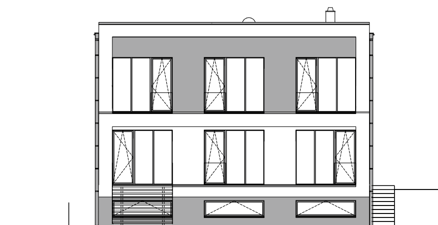
Jižní pohled | Southern view
